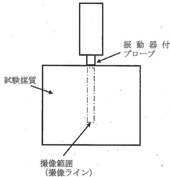
図5 伝搬速度、弾性率計測の模式図(例)
